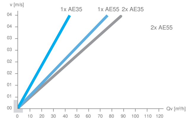
壓損作為流量率的函數
